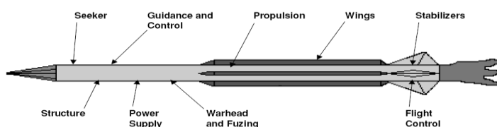
شکل ۱.۰ قسمت‌های مختلف یک موشک تاکتیکی.
